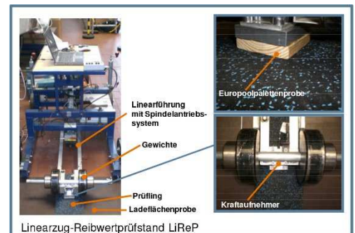
Linearzug-Reibwertprüfstand LiReP
