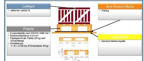
simuliertes Prüfszenario
