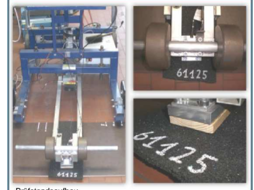
Prüfstands Aufbau
